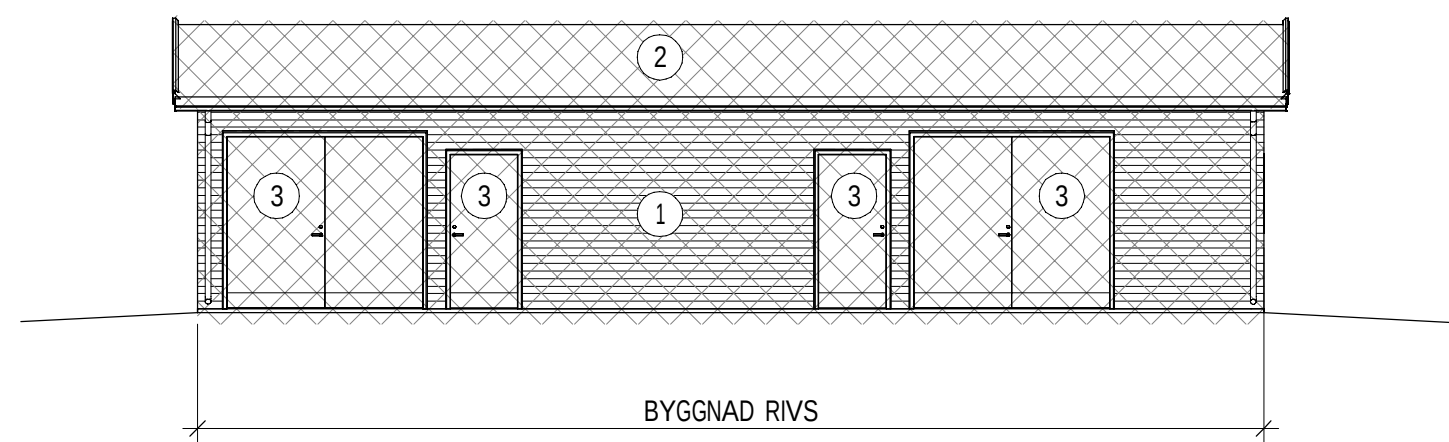
FÖRRÅD - FASAD MOT SYDVÄST 1 : 100
