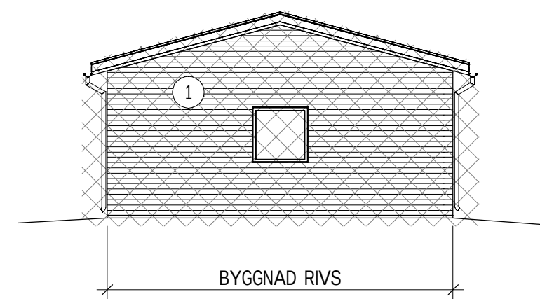
FÖRRÅD - FASAD MOT SYDÖST 1 : 100
