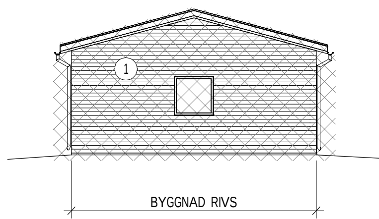
FÖRRÅD - FASAD MOT NORDVÄST 1 : 100
