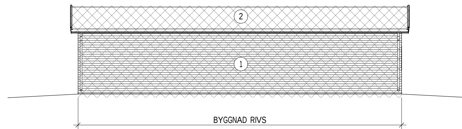
FÖRRÅD - FASAD MOT NORDÖST 1 : 100
